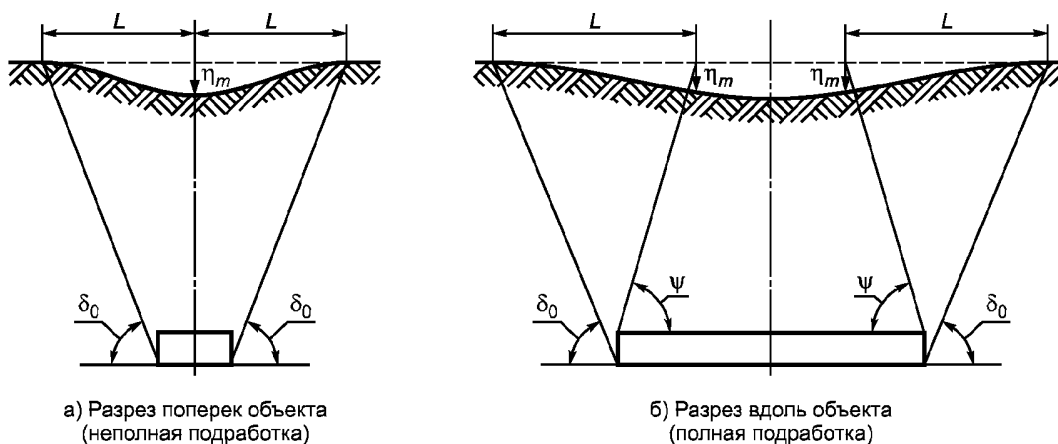
Рисунок С.1 — Основные параметры мульды сдвижения
