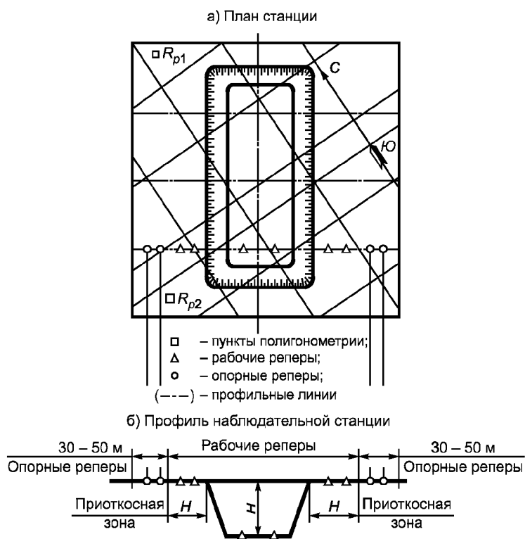
Рисунок У.2 — Схема к составлению проекта размещения реперов при открытом способе строительства подземного сооружения
